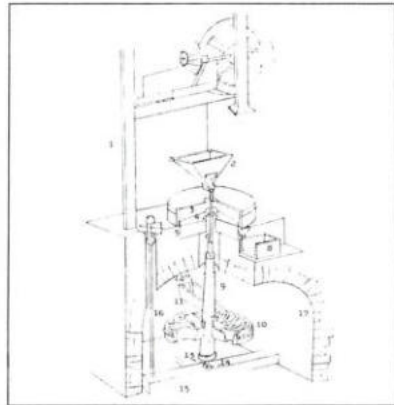
CROQUIS DELS MECANISMES DEL MOLÍ FARINER. LES PECES PRINCIPALS SÓN: LA CABRA (1); LA GRONSA (2); LA MOLA VOLANDERA (3); LA NAÏLLA (4); LA MOLA SOTANA (5); EL COLL-FERRO (6); EL FARINAL (7); LA FARNERA (8); L'ARBRE (9); EL RODET (10); LA CANAL (11); LA PALETA (12); L'AGULLA (13); EL DAU (14); EL BANC (15); EL TEMPLADOR (16); LA CACAU (17).
